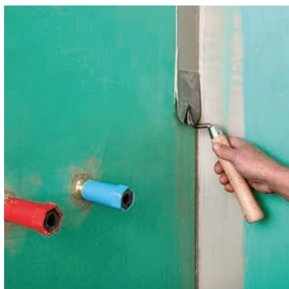
Před realizací detailů (napojení stěna-podlaha a stěna-stěna) nanést dostatečné množství hydroizolačního materiálu.
